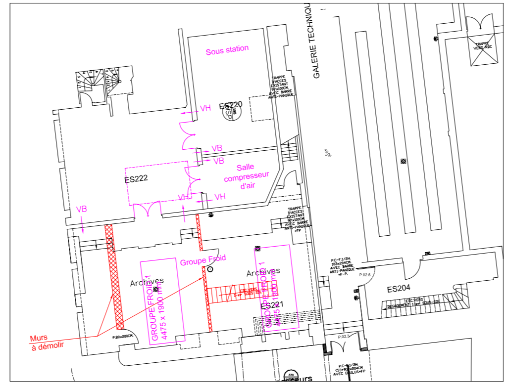
Zoom sur L.T. (groupes froids + sous-station chaufferie)
